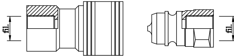
Quick coupling ball Innesti rapidi a sfera
