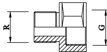
Male adaptor. Raccordo di riduzione.
