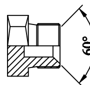
Plugs male Tappi maschio
