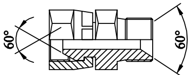
Adaptors female swivel Adattatori maschio fisso femmina girevole
